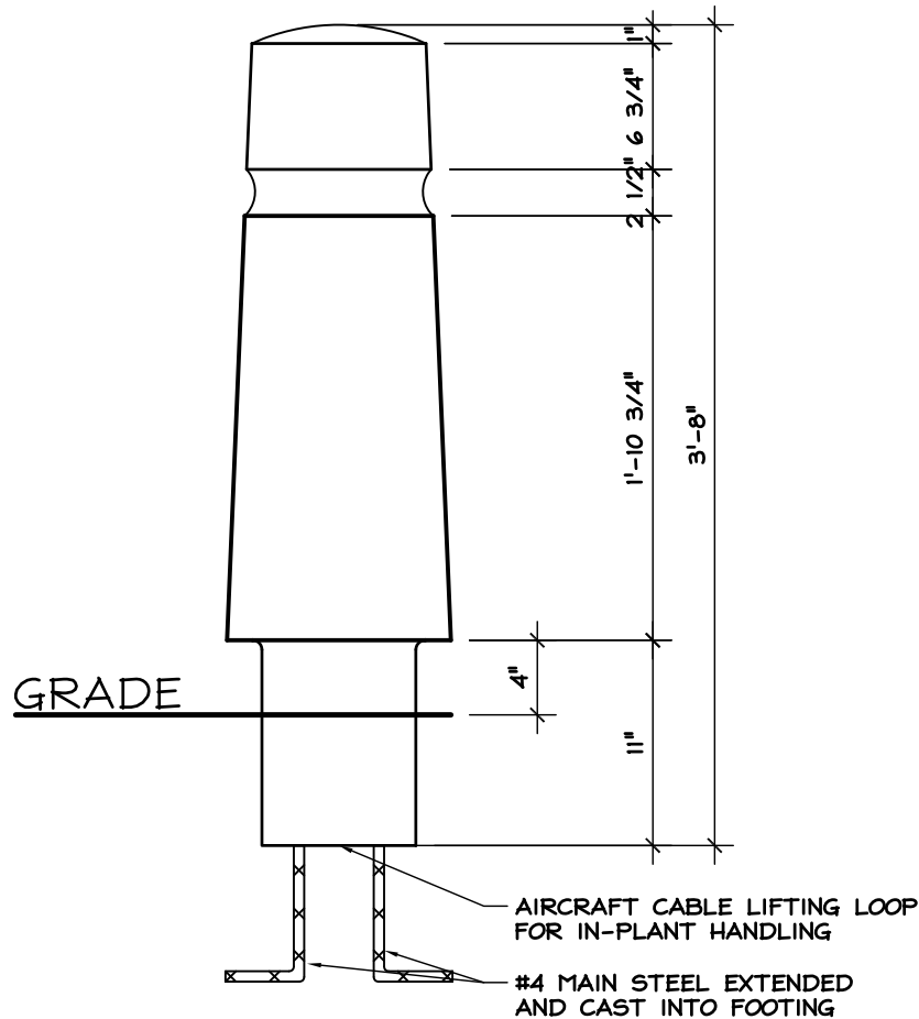
ELEVATION
