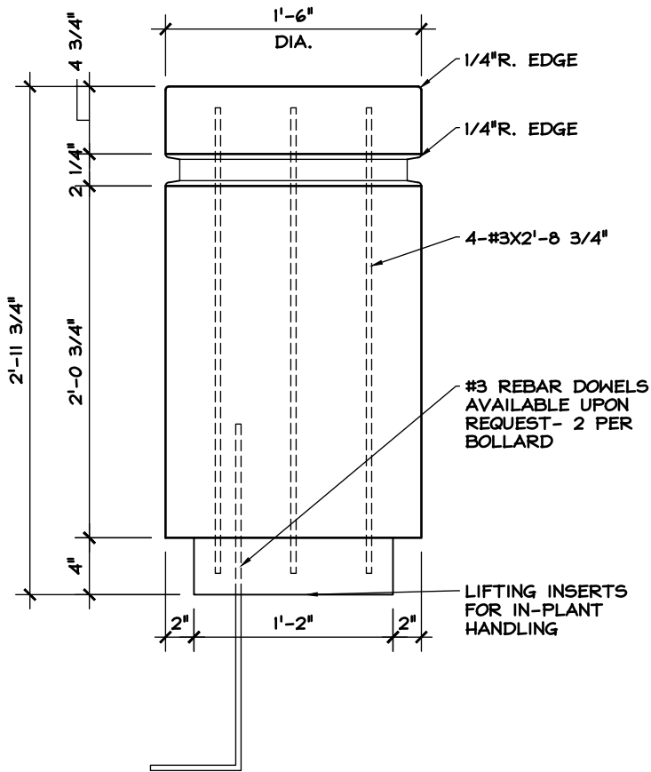
ELEVATION
