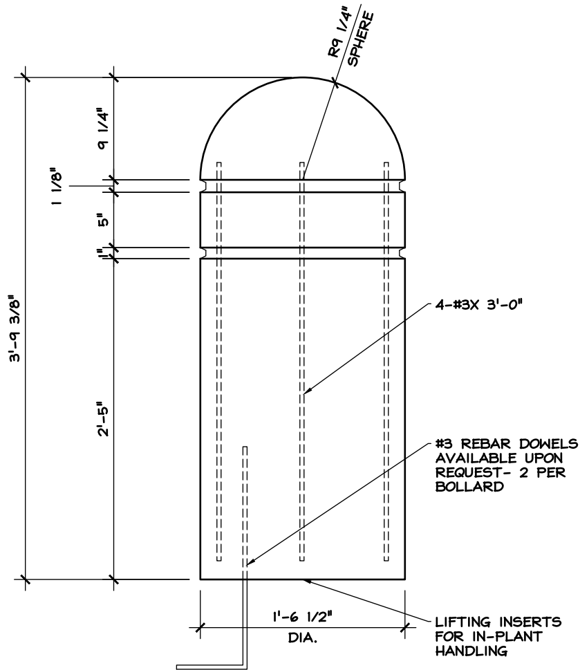
ELEVATION
